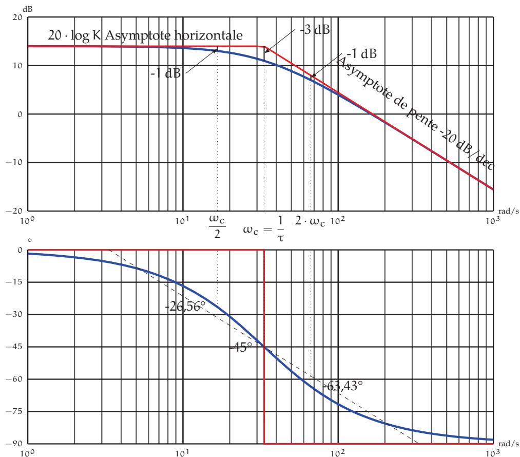
FIGURE 6.4 – Diagrammes de Bode - Système du 1 er ordre
