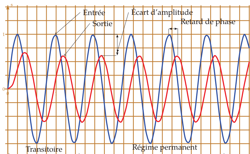
FIGURE 6.2 – Réponse fréquentielle
