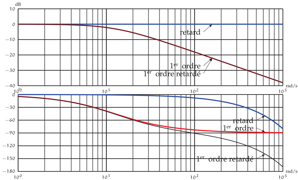
FIGURE 6.10 – Diagrammes de Bode - Influence d'un retard
