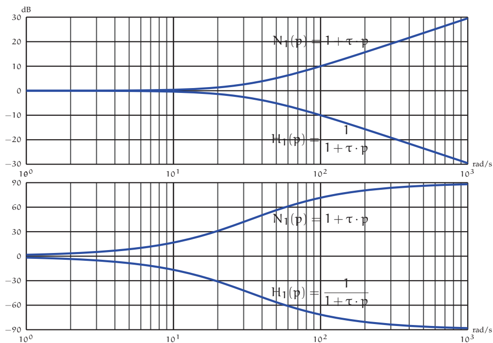
FIGURE 6.5 – Diagrammes de Bode - 1 er ordre au numérateur
