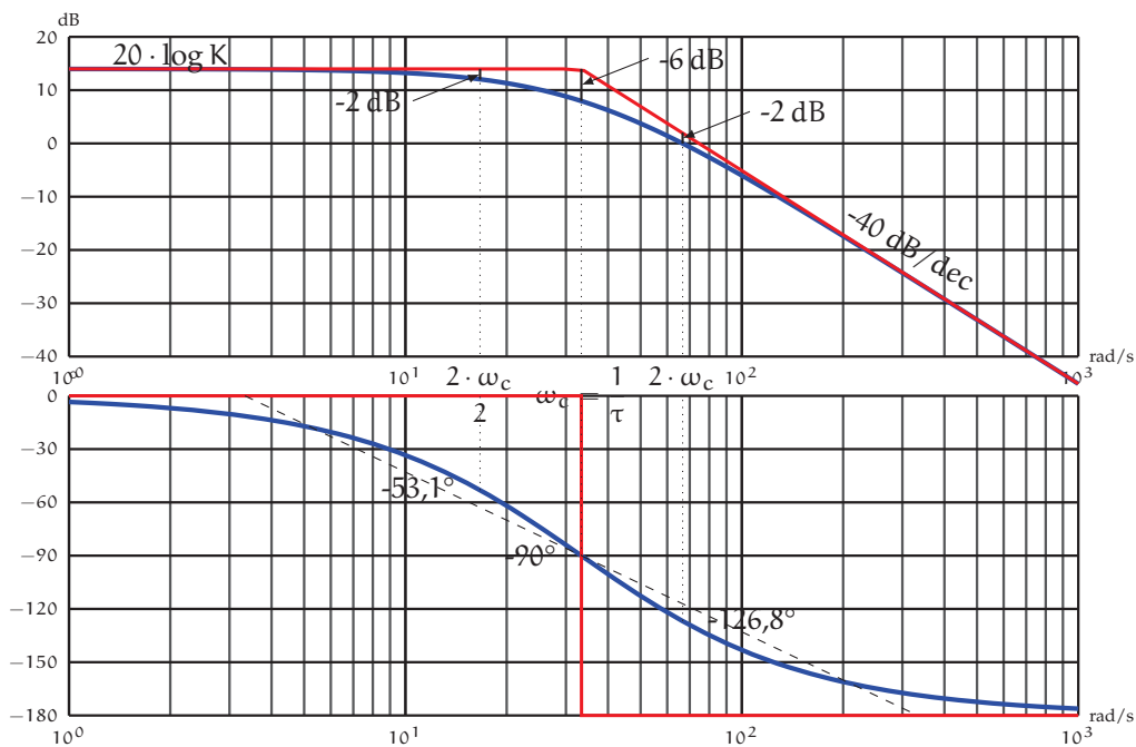
FIGURE 6.8 – Diagrammes de Bode 2 nd ordre - 1 racine double
