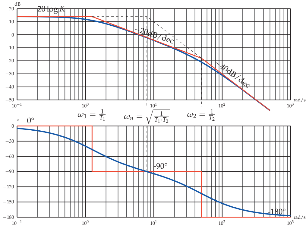
FIGURE 6.7. – Diagrammes de Bode 2 nd ordre - 2 racines réelles
