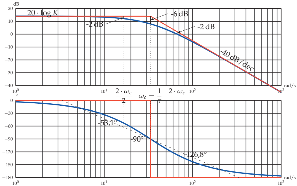
FIGURE 6.8. – Diagrammes de Bode 2 nd ordre - 1 racine double
