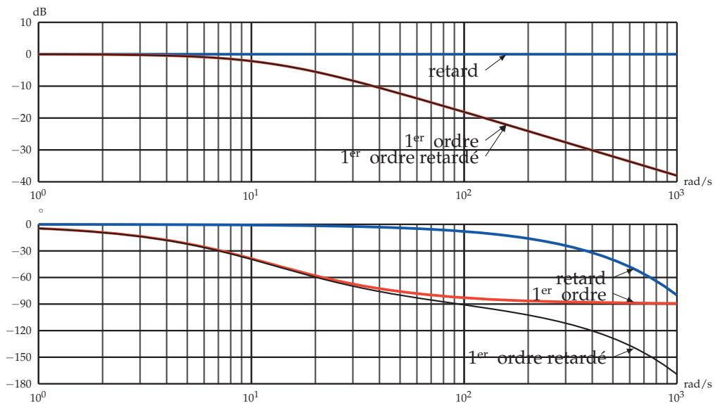
FIGURE 6.10. – Diagrammes de Bode - Influence d'un retard
