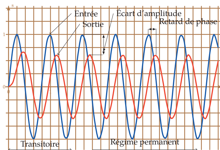
FIGURE 6.2. – Réponse fréquentielle
