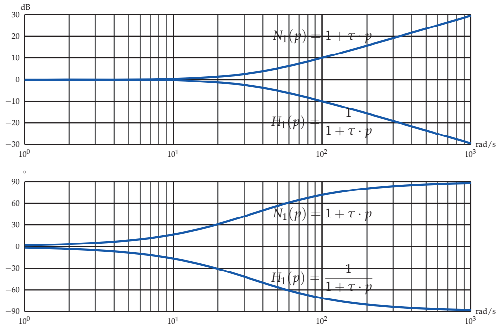
FIGURE 6.5. – Diagrammes de Bode - 1 er ordre au numérateur
