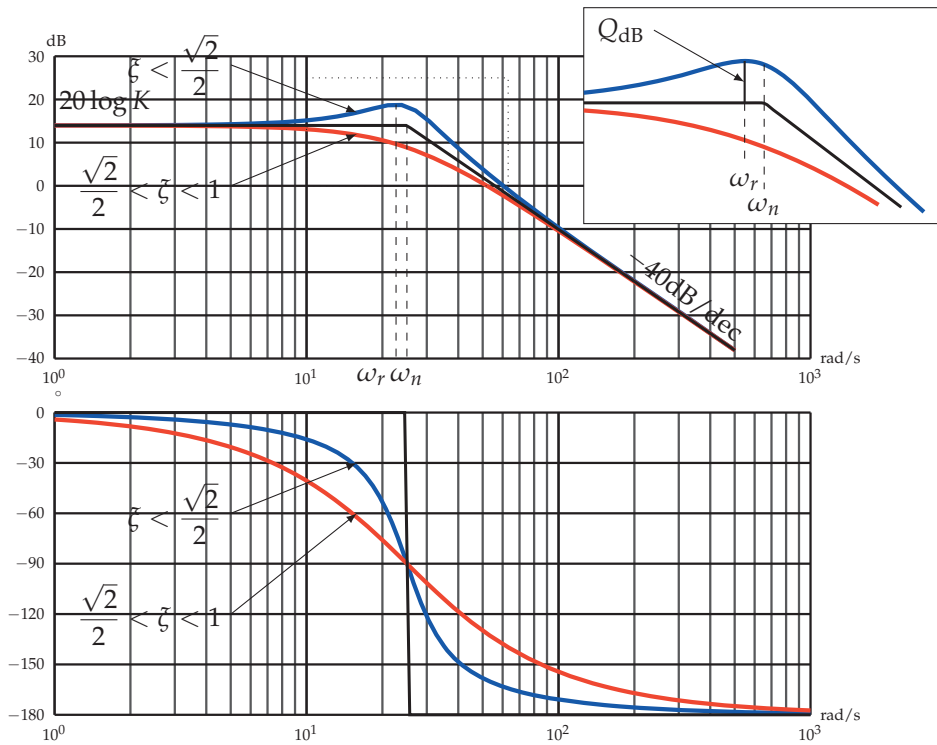
FIGURE 6.6. – Diagrammes de Bode 2 nd ordre - 2 racines complexes
