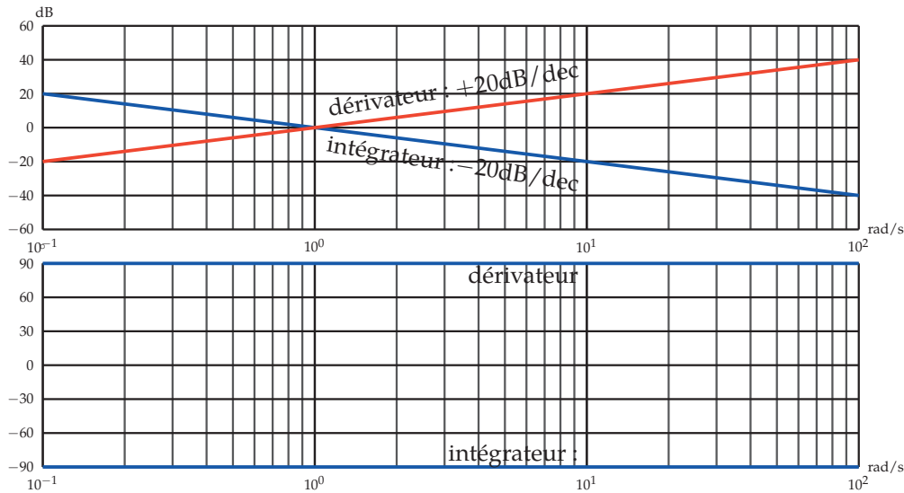
FIGURE 6.9. – Diagrammes de Bode - Intégrateur - Dérivateur
