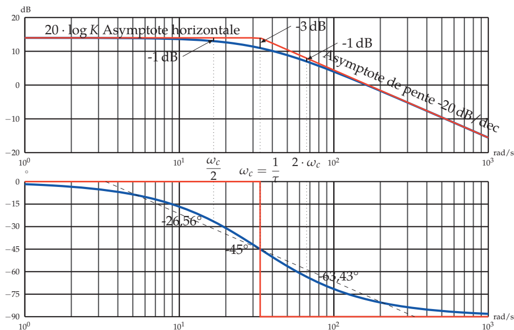
FIGURE 6.4. – Diagrammes de Bode - système du 1 er ordre
