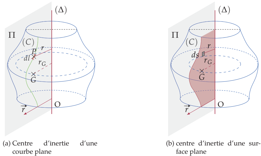
FIGURE 2.2. – Théorèmes de Guldin
