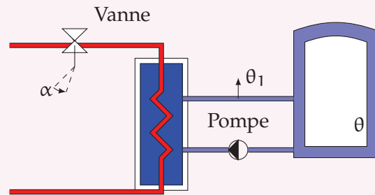
FIGURE 3.12 – Échangeur thermique
