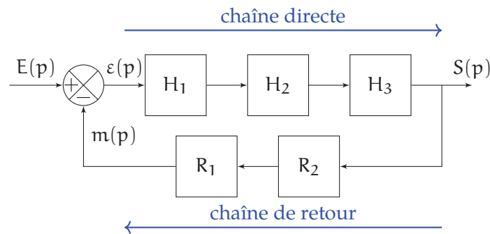
FIGURE 4.3 – forme générale
