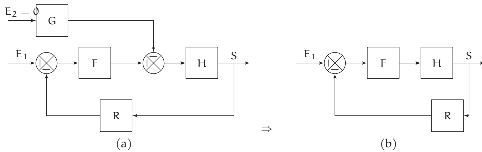
FIGURE 4.12 – Sschéma-bloc
