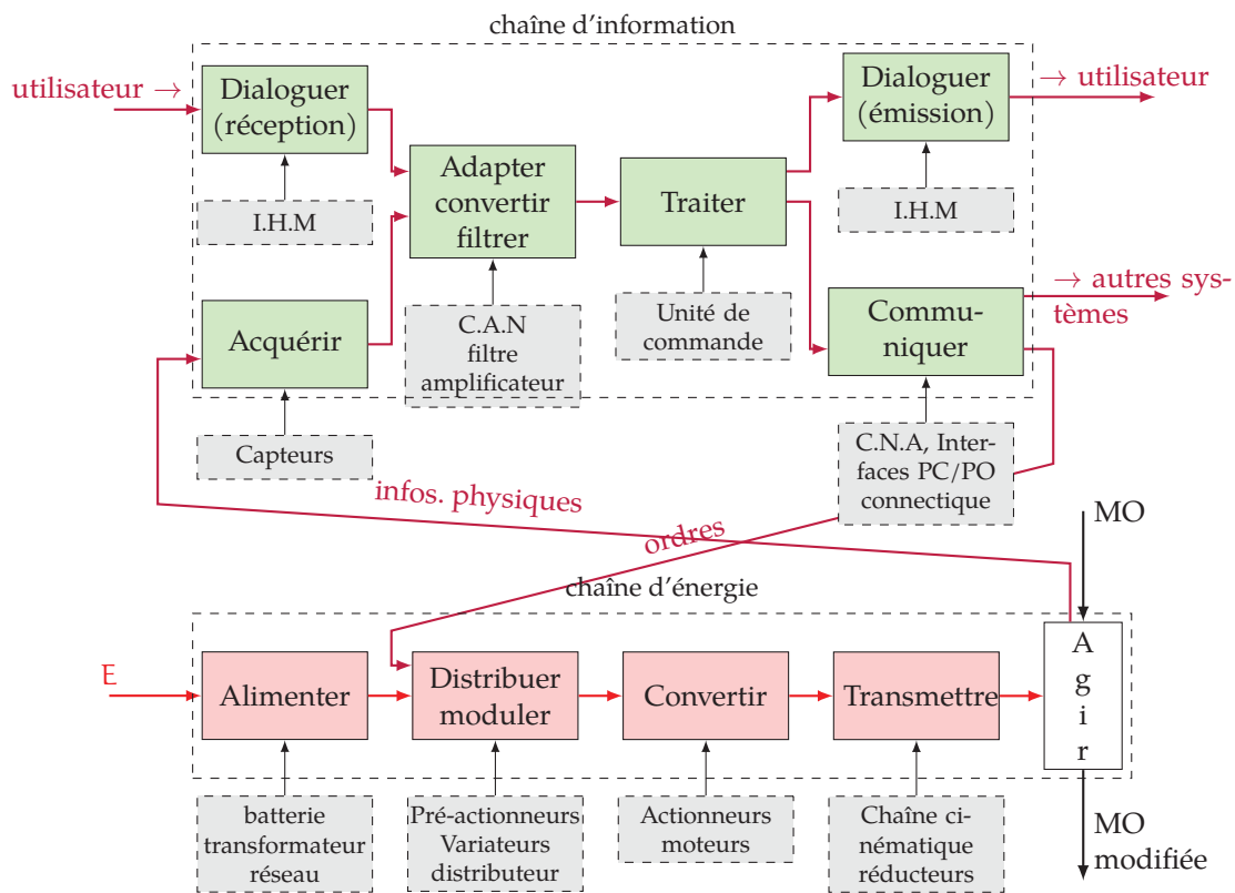
FIGURE 1.19 – Description fonctionnelles des chaînes d'information et d'énergie
