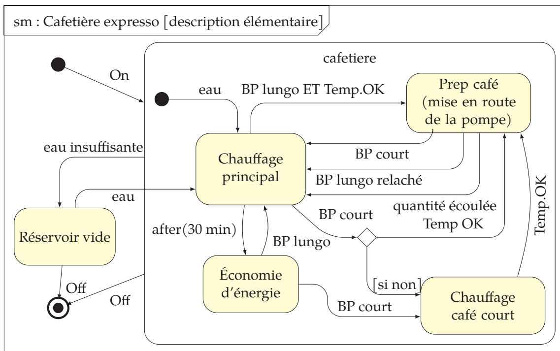
FIGURE 1.14 – Diagramme états-transitions de la cafetière expresso [description élémentaire]
