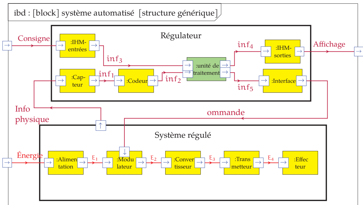
FIGURE 1.21 – Structure générique d'un système automatisé - Détails
