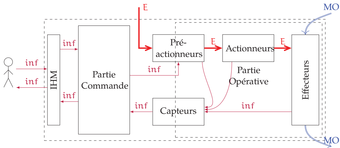
FIGURE 1.18 – Décomposition structurelle d'un système automatisé
