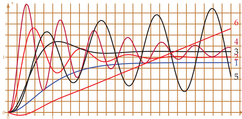
FIGURE 2.7 – Stabilité
