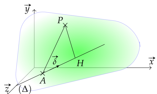
FIGURE 2.3 – Moment d'inertie
